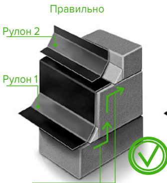
Смена направления укладки
