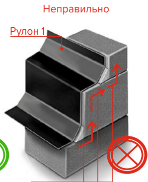
Смена направления укладки
