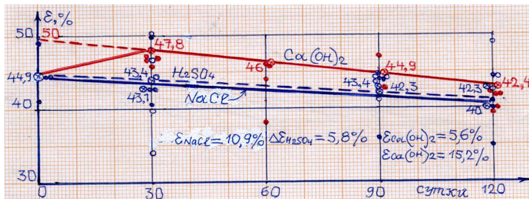
Рисунок 1 - Изменение деформативности наплавляемого рулонного материала марки Техноэласт П ЭПП при воздействии химических реагентов
